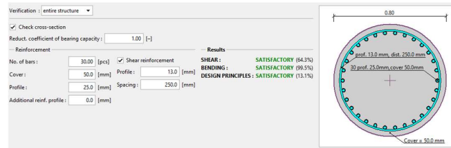
Gambar 14. Tulangan kombinasi Ekstrim 1
